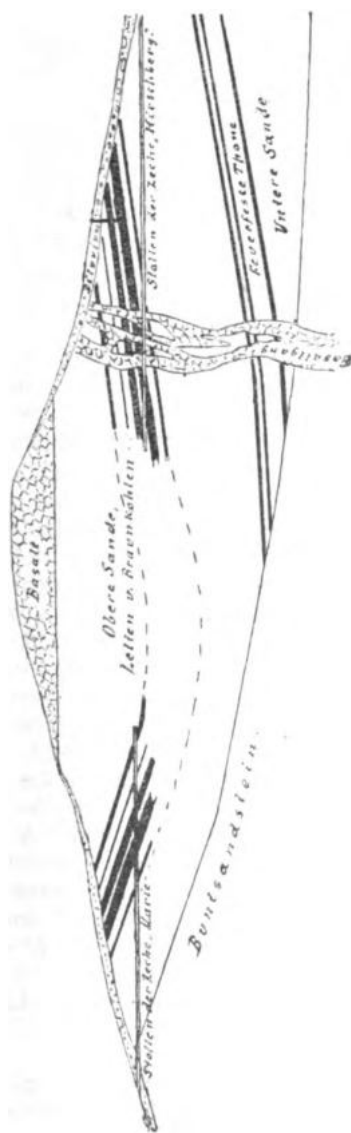
Profil des Hirschberges. Nach Uhlemaun's „Braunkohlenlagerstätten“. Abhandlung der Königl. preuss. geologischen Landesanstalt. Berlin bei Schropp. Maassstab 1 : 10 000.
