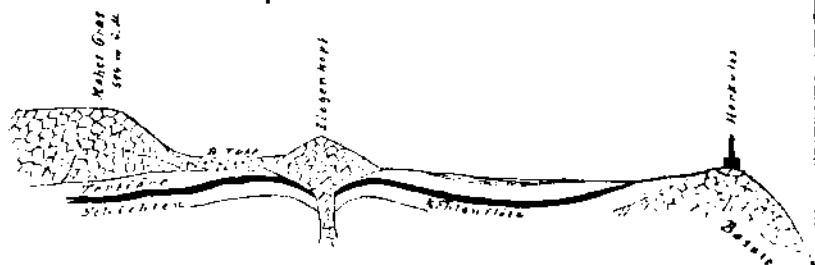
Profil des Habichtswaldes (schematisch dargestellt.)
