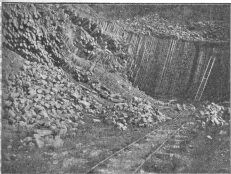
Untere Abtheilung des Basaltbruches bei Blitzenrod.
